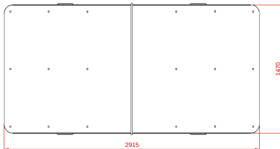
PLANTA
