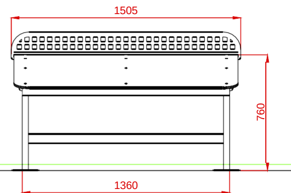
PERFIL
