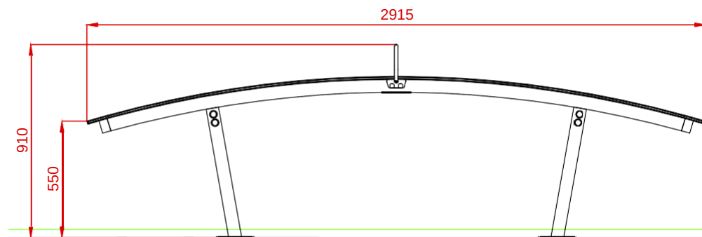
ALZADO
